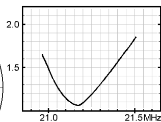
VSWR
