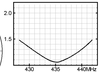
VSWR特性
