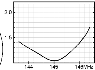
VSWR 特性
